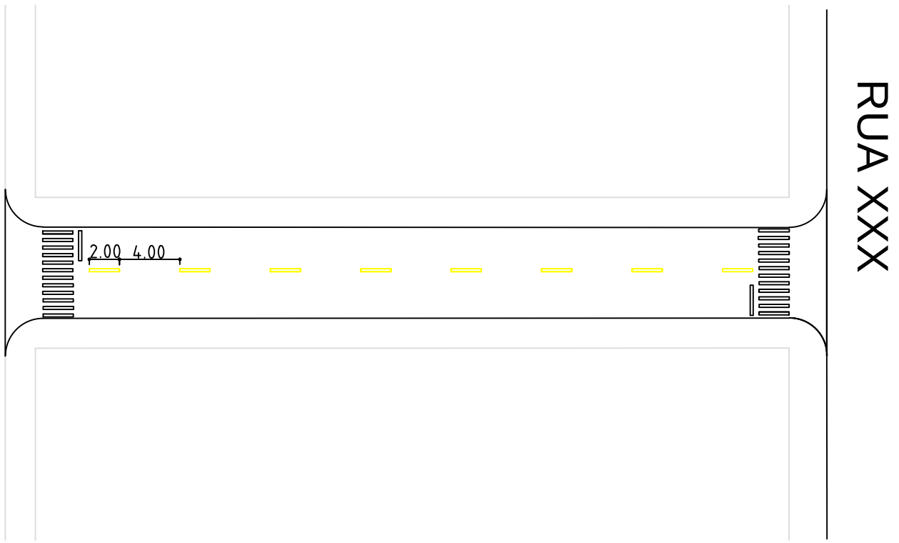
DETALHE FAIXA DIVISÃO DE FLUXO Escala: 1:50
